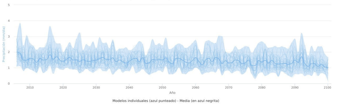
Figura 3.- Projecció de precipitació diària a les Illes Balears per a l'escenari d'emissions RCP4.5 (dalt) i RCP8.5 (baix) (Font: visor AdapteCCa).
