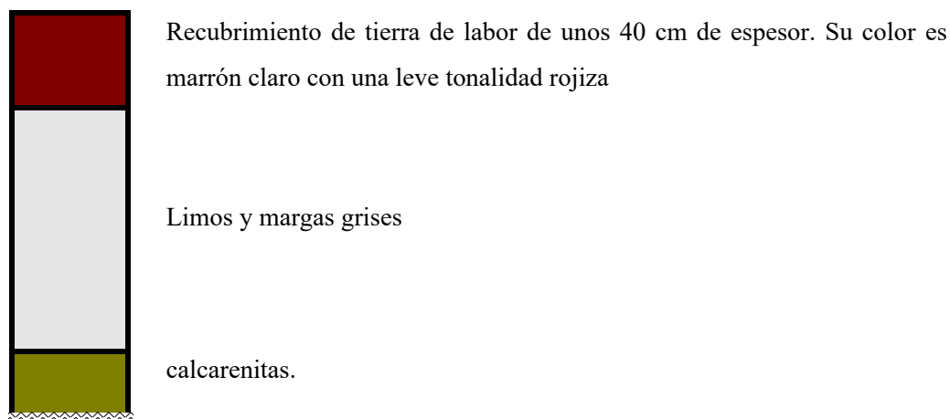
Figura 6: Columna estratigráfica.
