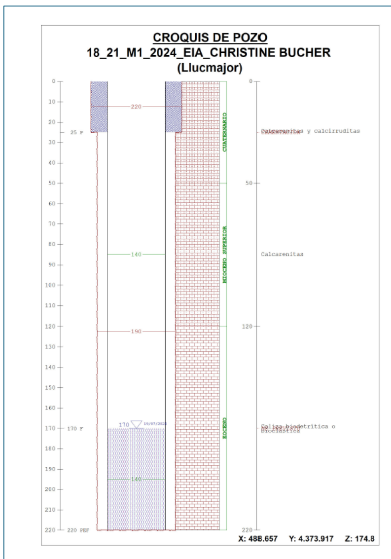
Figura 8: corte estratigráfico
