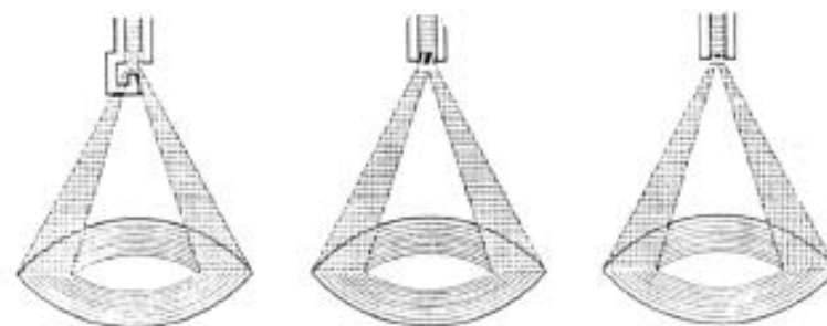
Fig. 14.—Esquema de boquillas de cono hueco.
