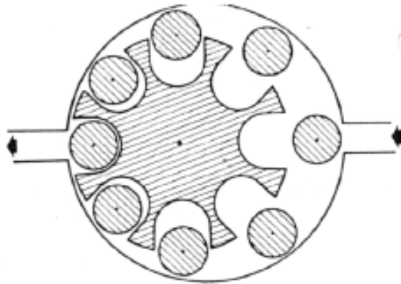
Fig. 9.—Esquema de una bomba de rodillos.
