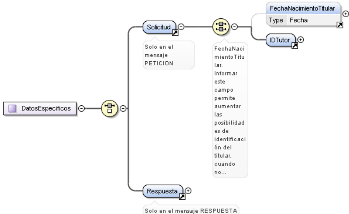
Figura 5. Esquema del node <DatosEspecificos> en una petició via el Recubrimiento WS.
