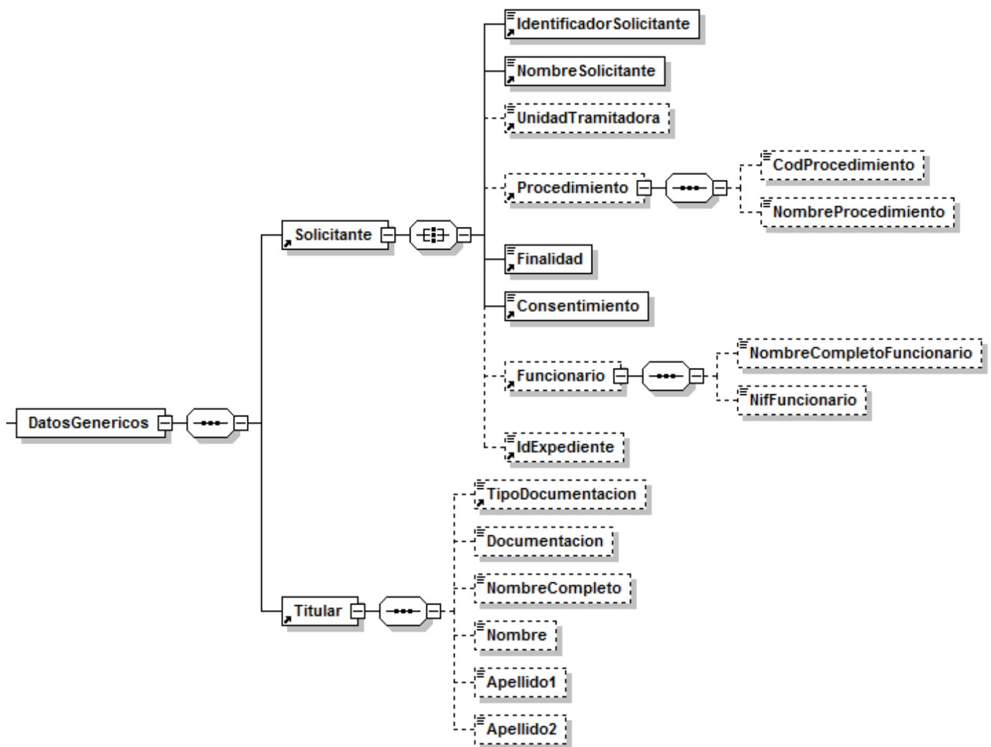
Figura 4. Esquema del node <DatosGenericos> en una petició via el Recubrimiento WS.
