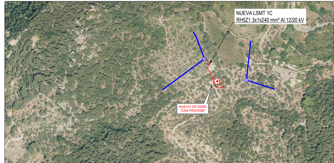
PLANO DE EMPLAZAMIENTO ESC: 1:5000
