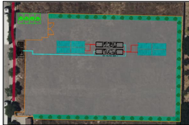
Imagen 8 Implantación general
