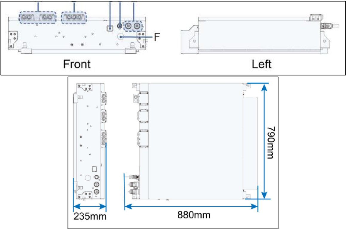
Imagen 13: Detalle de los inversores.
