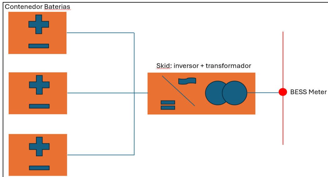
Imagen 11: Esquema sistema inversor centralizado.
