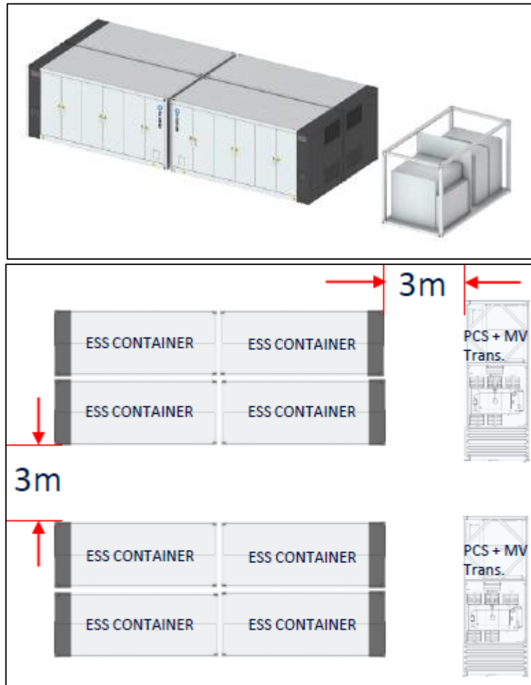
Imagen 19: Distancias mínimas para el mantenimiento.
