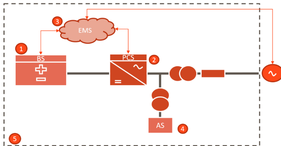
Imagen 9: Configuración típica de un sistema BESS
