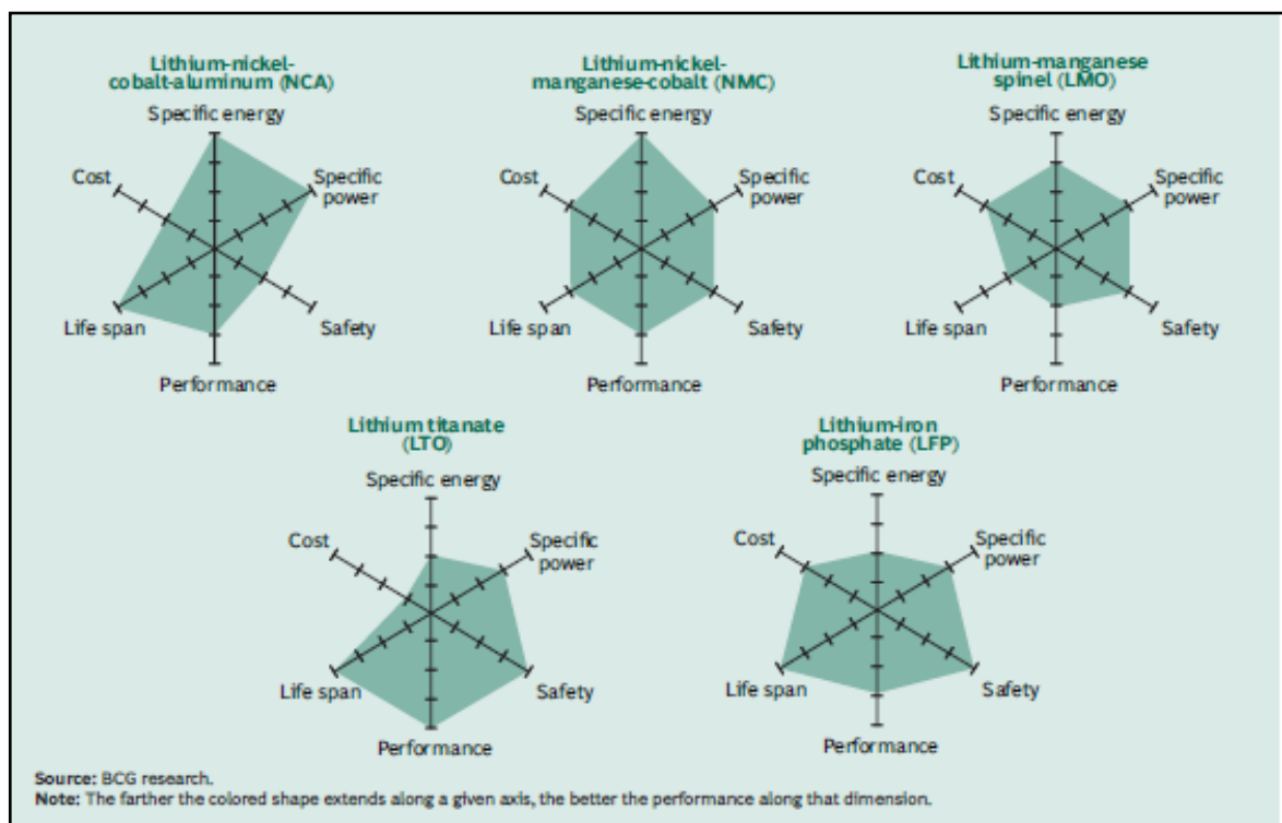
Imagen 8.. Principales características de Tecnologías Ion-Litio
