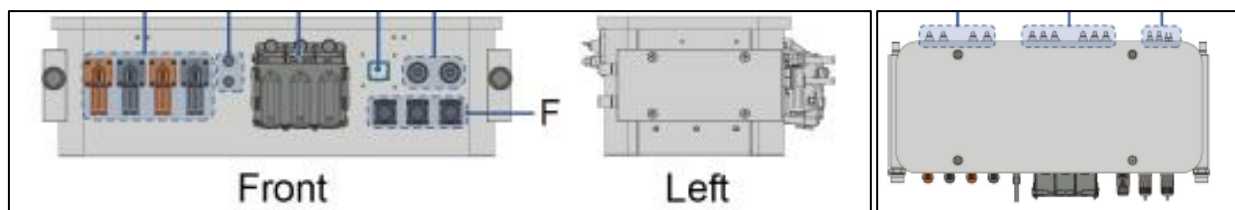
Imagen 14: Detalle de las cajas de terminales de protección.
