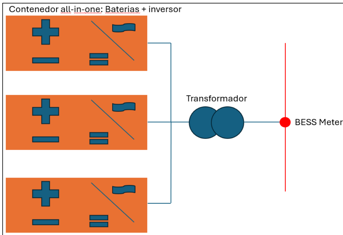
Imagen 10: Esquema sistema all-in-one.
