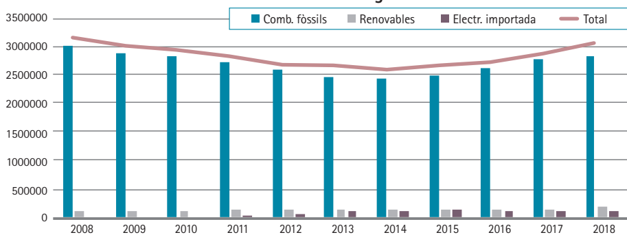
Gràfic I-11.72. Variació interanual consum energètic 2008-2018
