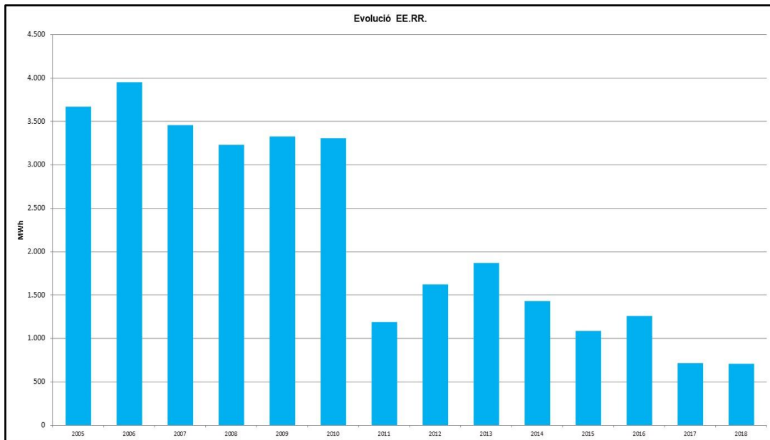
Gràfic 10. Evolució de l'energia generada amb renovables (MWh)
