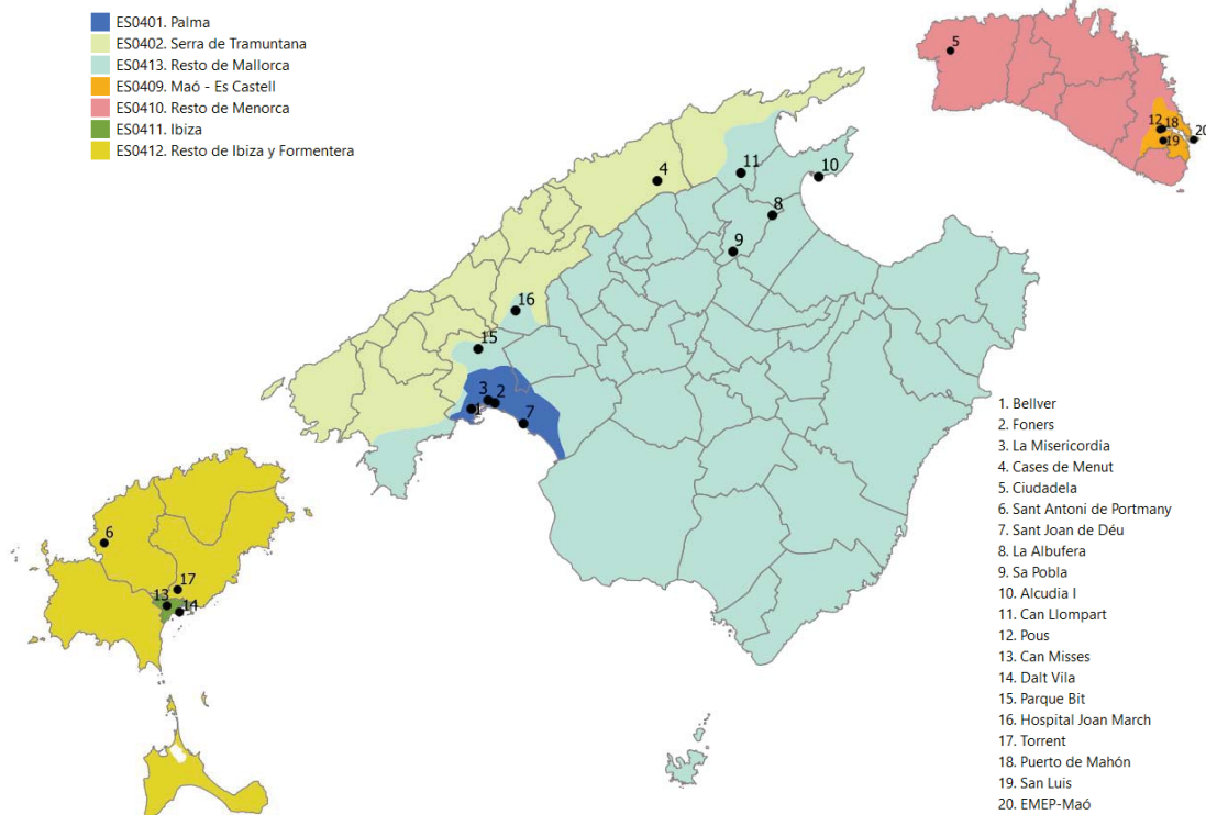
Figura 1. Zonificación para la evaluación de la calidad del aire en las Islas Baleares. Fuente: elaboración propia a partir de cartografía del MITECO y de información perteneciente al Govern Illes Balears.
