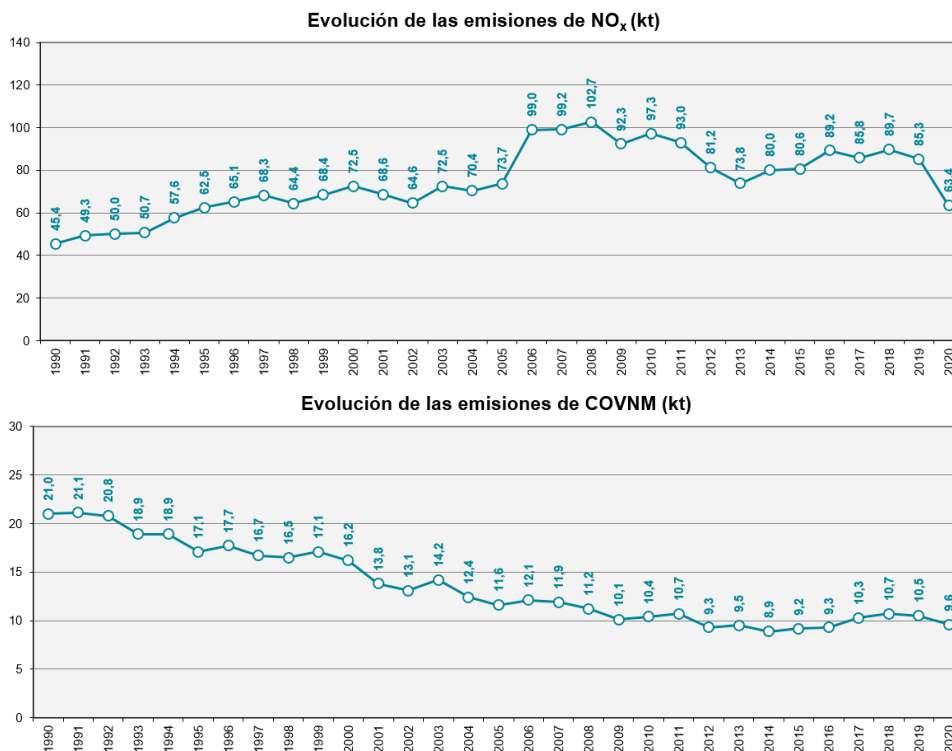
Figura 24. Evolución de las emisiones de precursores (Balears, 1990-2020). Fuente: Servicio de Cambio Climático y Atmósfera de la Dirección General de Energía y Cambio Climático de las Islas Balears.
