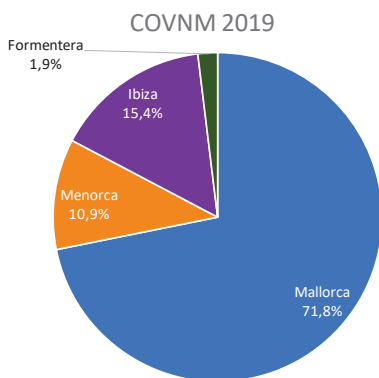
Figura 29. Distribución porcentual de emisiones de COVNM por islas (Balears, 2019).
