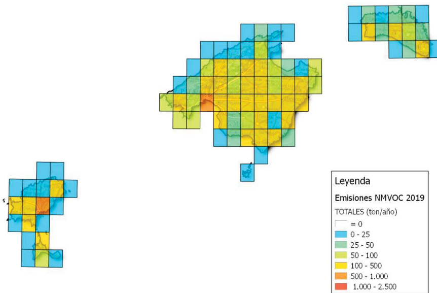
Figura 31. Distribución espacial de emisiones de COVNM (Balears, 2019).
