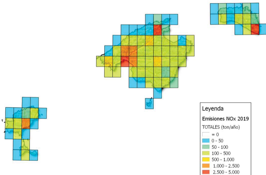
Figura 30. Distribución espacial de emisiones de NOx (Baleares, 2019).
