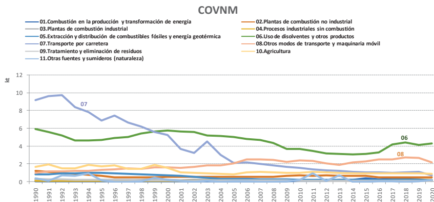
Figura 25. Evolución de emisiones sectoriales de precursores (Balears, 1990-2020).
