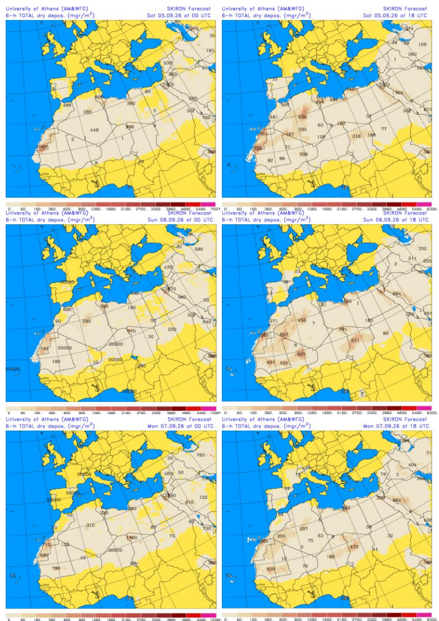
Depósito seco de polvo (mg/m 2 ) predicho por el modelo SKIRON para los días 5, 6 y 7 de septiembre de 2026 a las 00 y 18 UTC © Universidad de Atenas.
