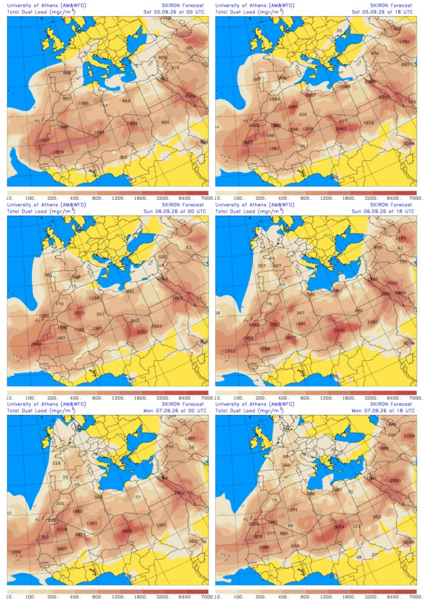
Carga total de polvo (mg/m²) predicha por el modelo SKIRON para los días 5, 6 y 7 de septiembre de 2026 a las 00 y 18 UTC © Universidad de Atenas.
