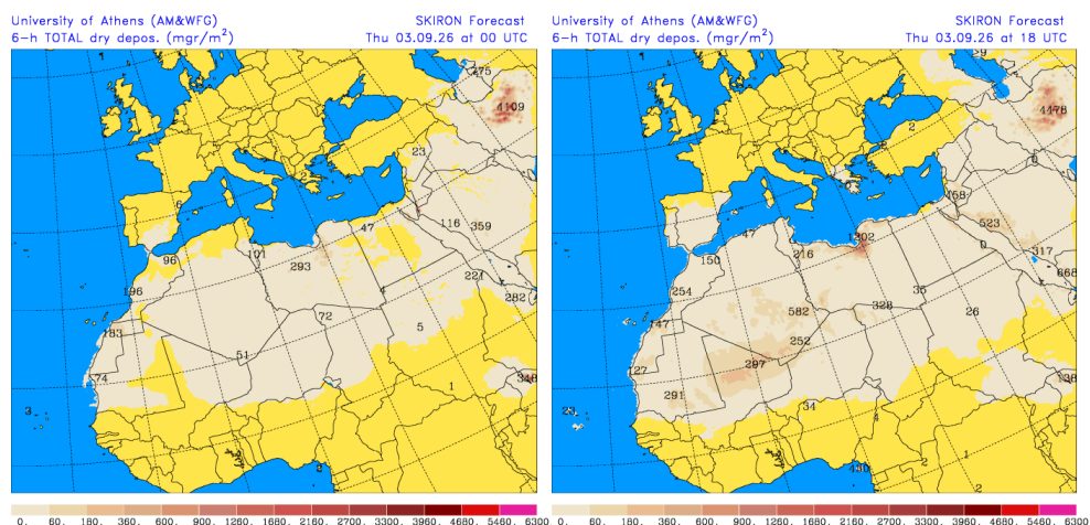
Depósito seco de polvo ( \text{mg}/\text{m}^2 ) predicho por el modelo SKIRON para el día 3 de septiembre de 2026 a las 00 y 18 UTC © Universidad de Atenas.
