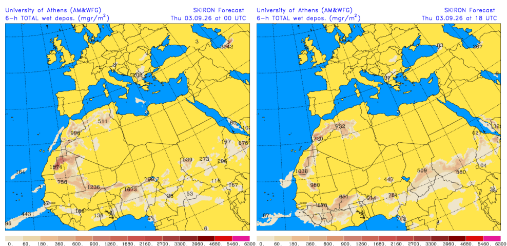
Depósito húmedo de polvo ( \text{mg}/\text{m}^2 ) predicho por el modelo SKIRON para el día 3 de septiembre de 2026 a las 00 y 18 UTC © Universidad de Atenas.
