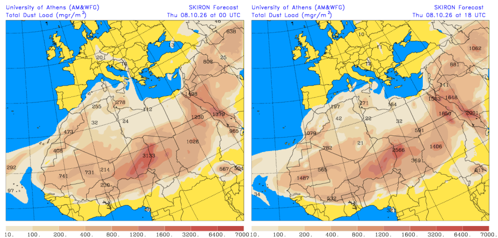
Carga total de polvo (mg/m 2 ) predicha por el modelo SKIRON para el día 8 de octubre de 2026 a las 00 y 18 UTC © Universidad de Atenas.
