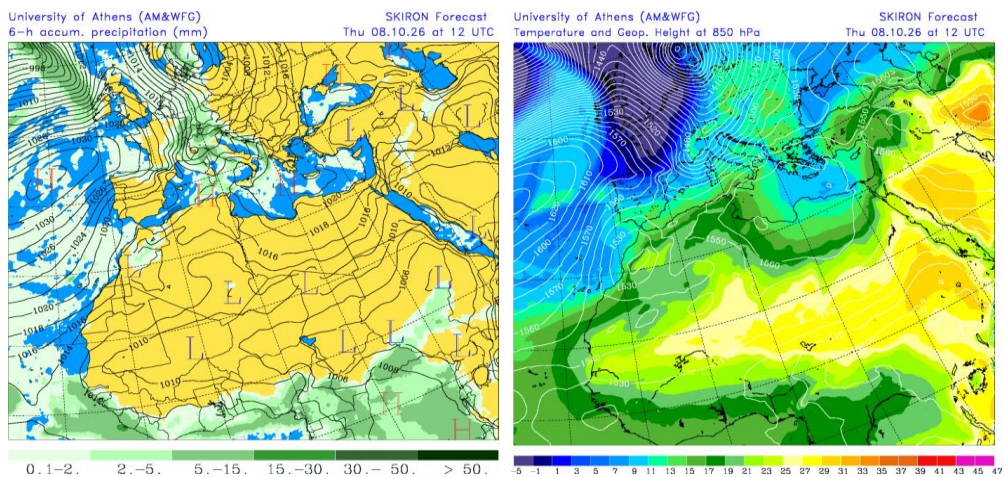
Precipitación acumulada (mm) y presión a nivel del mar (hPa) (izquierda) y campo de temperaturas (°C) y de altura geopotencial a 850 hPa (derecha) previsto por el modelo SKIRON para el día 8 de octubre de 2026 a las 12 UTC © Universidad de Atenas.
