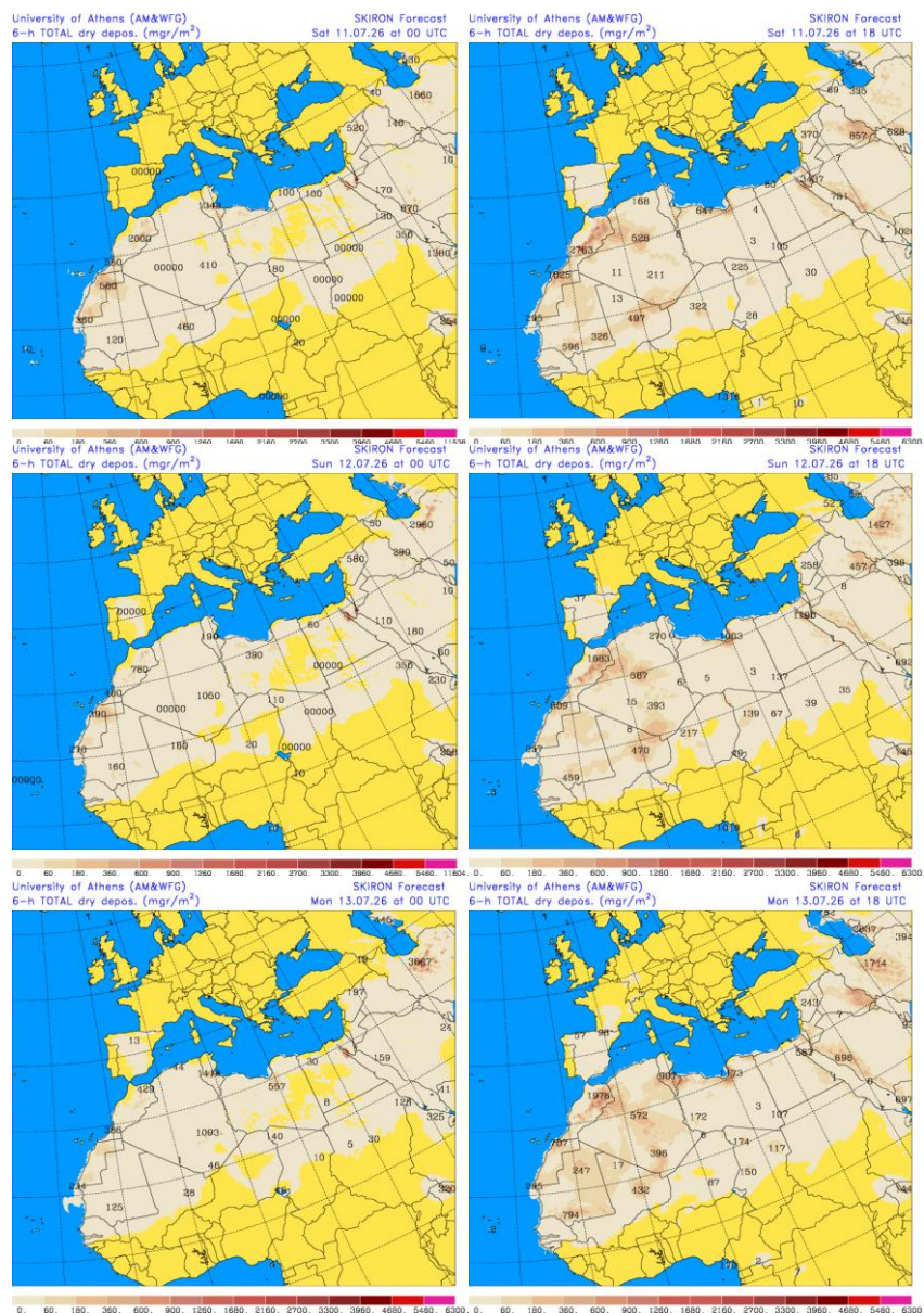
Depósito seco de polvo (mg/m 2 ) predicho por el modelo SKIRON para los días 11, 12 y 13 de julio de 2026 a las 00 y 18 UTC © Universidad de Atenas.
