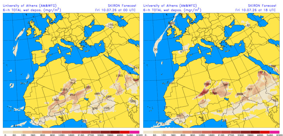
Depósito húmedo de polvo (mg/m 2 ) predicho por el modelo SKIRON para el día 10 de julio de 2026 a las 00 y 18 UTC © Universidad de Atenas.
