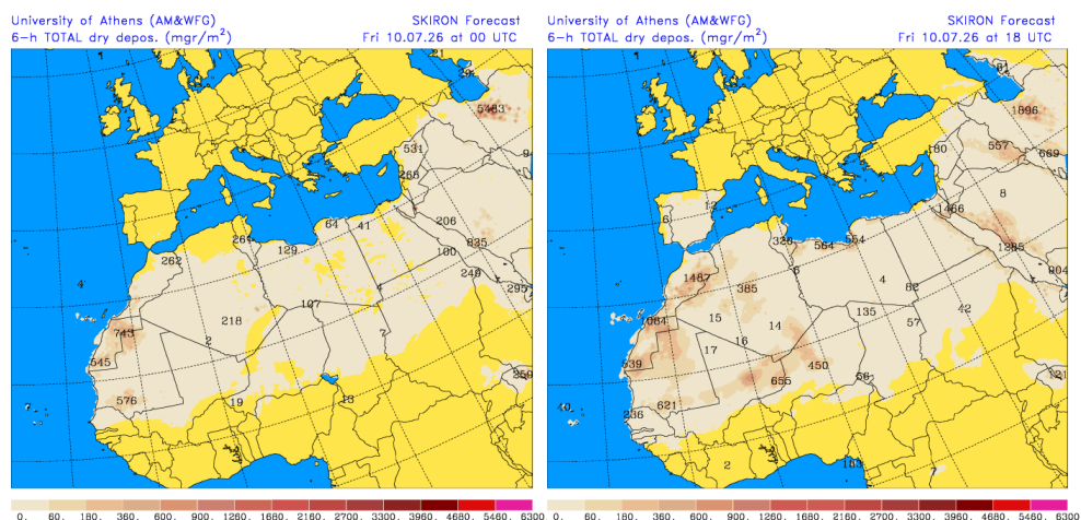
Depósito seco de polvo (mg/m 2 ) predicho por el modelo SKIRON para el día 10 de julio de 2026 a las 00 y 18 UTC © Universidad de Atenas.
