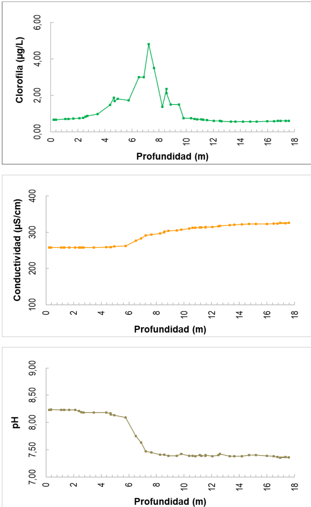
Figura 6: Gráficas de las variables ambientales obtenidas en los perfiles de profundidad en el embalse de Gorg Blau
