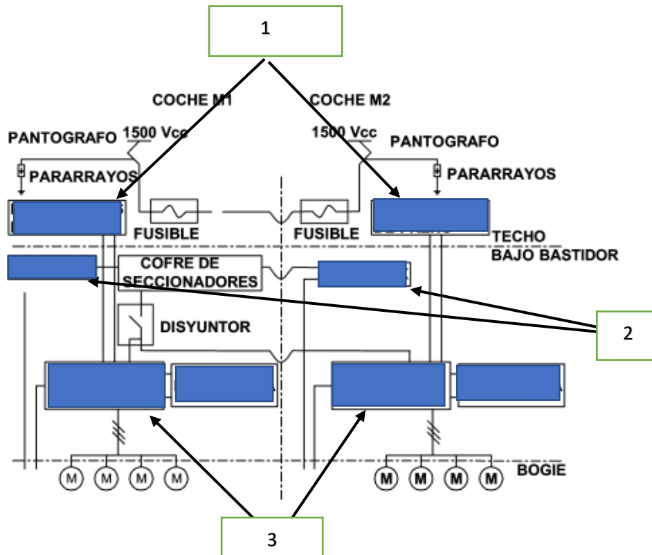
FIGURA 9. CIRCUITO ALTA TENSION 7100
