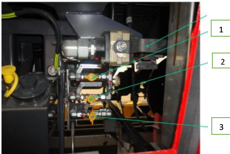
FIGURA 12. LLAVES AISLAMIENTO 8100
