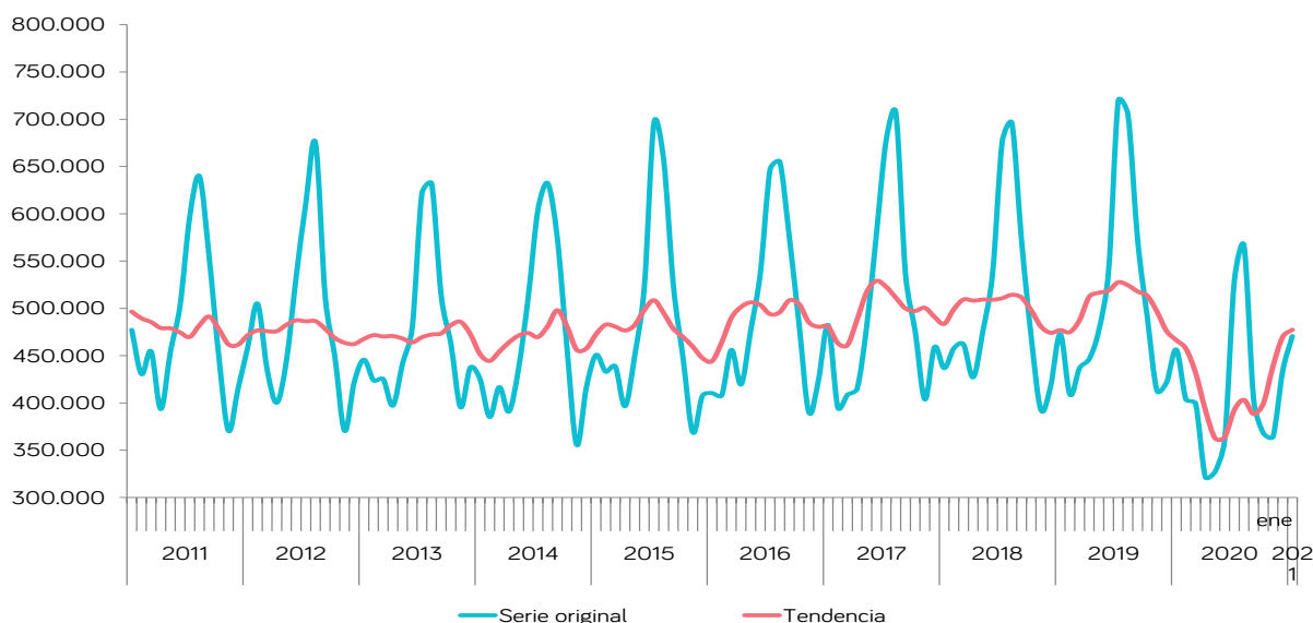
Gráfico 8. Energía eléctrica mensual demandada en las Islas Baleares (MWh)
