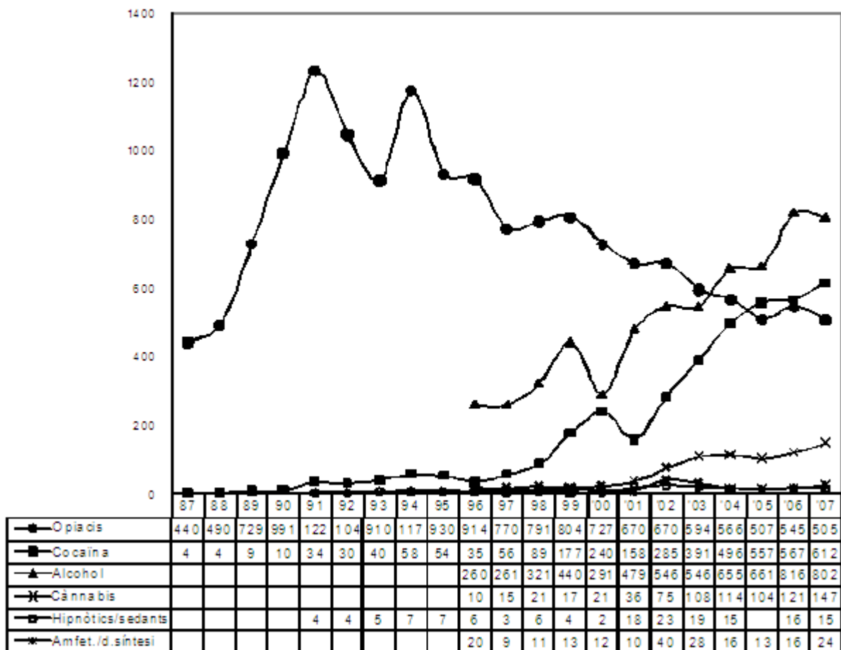
Gràfic 1. Evolució del nombre d'admissions per droga principal, 1987-2007
