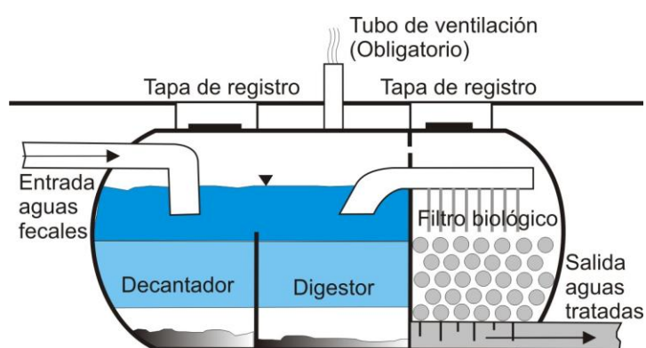
Figura 3. Fosa séptica con filtro percolador.
